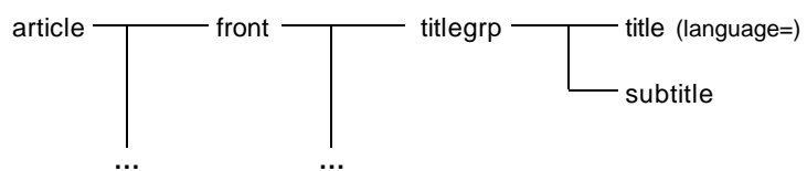
FIGURA 3 Diagrama do segmento do grupo de título da DTD SciELO Article
