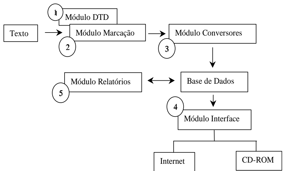
FIGURA 1 Diagrama de fluxo de dados entre os módulos da Metodologia SciELO
