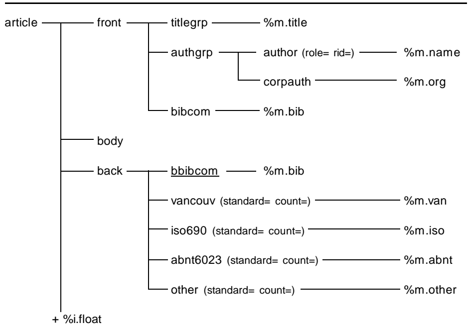
FIGURA 2 Estrutura geral da DTD SciELO Article para artigos de periódicos eletrônicos
